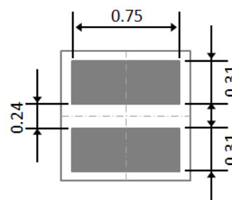
<PCB Land>
